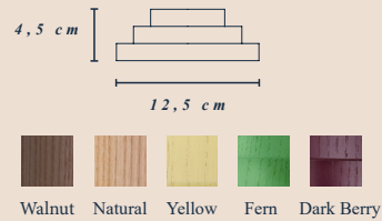
Pyramid
