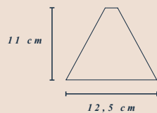
Cone
