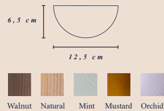
Moon
